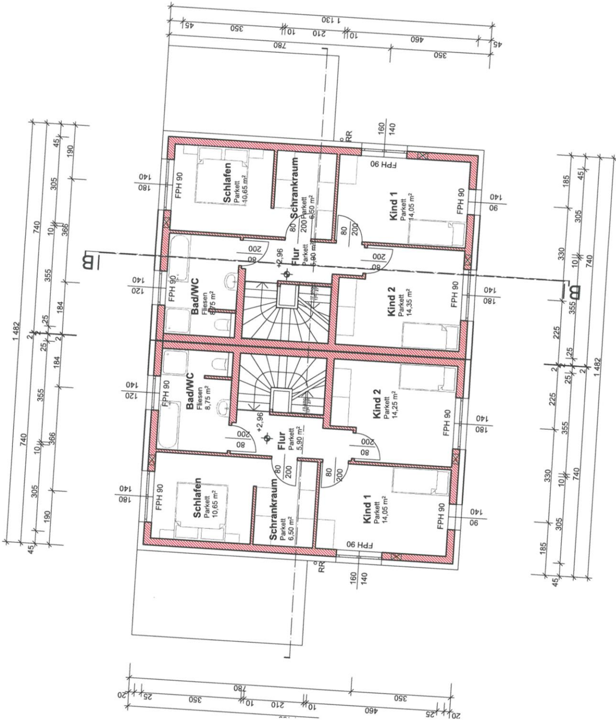
OBERGESCHOSS WNFL im OG: 60,10m² pro Doppelhaushälfte
