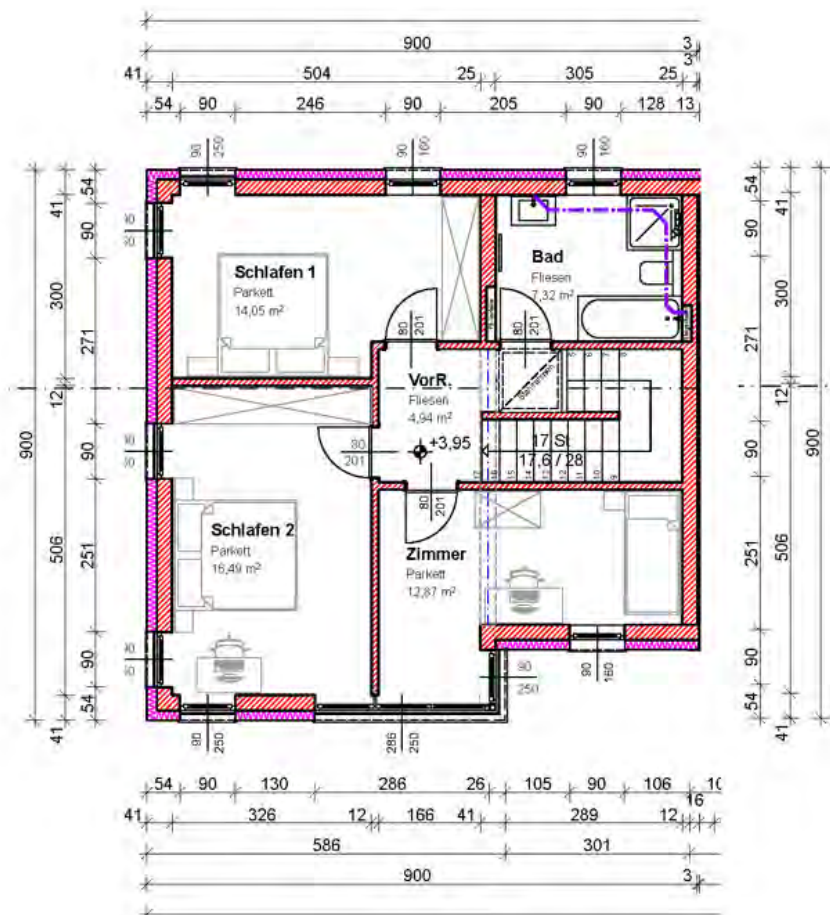
Grundriss Obergeschoss
