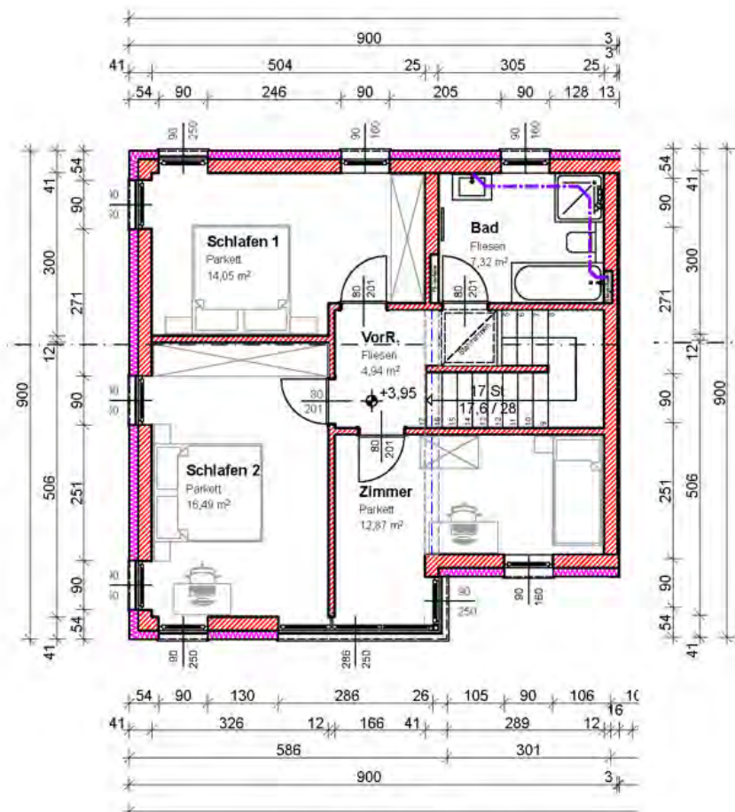
Grundriss Obergeschoss
