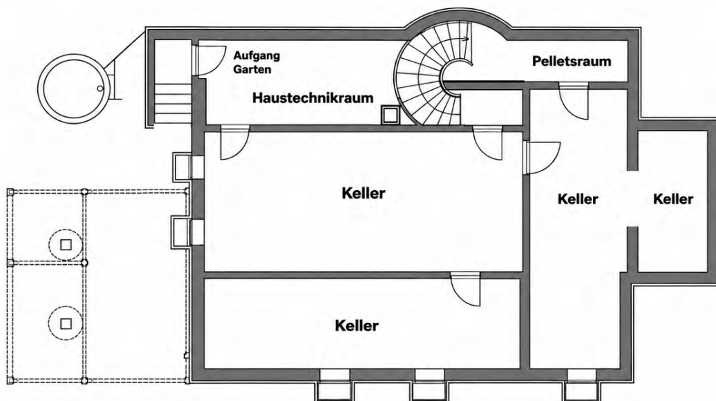
Grundriss_Keller
